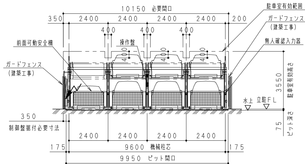
正面図
