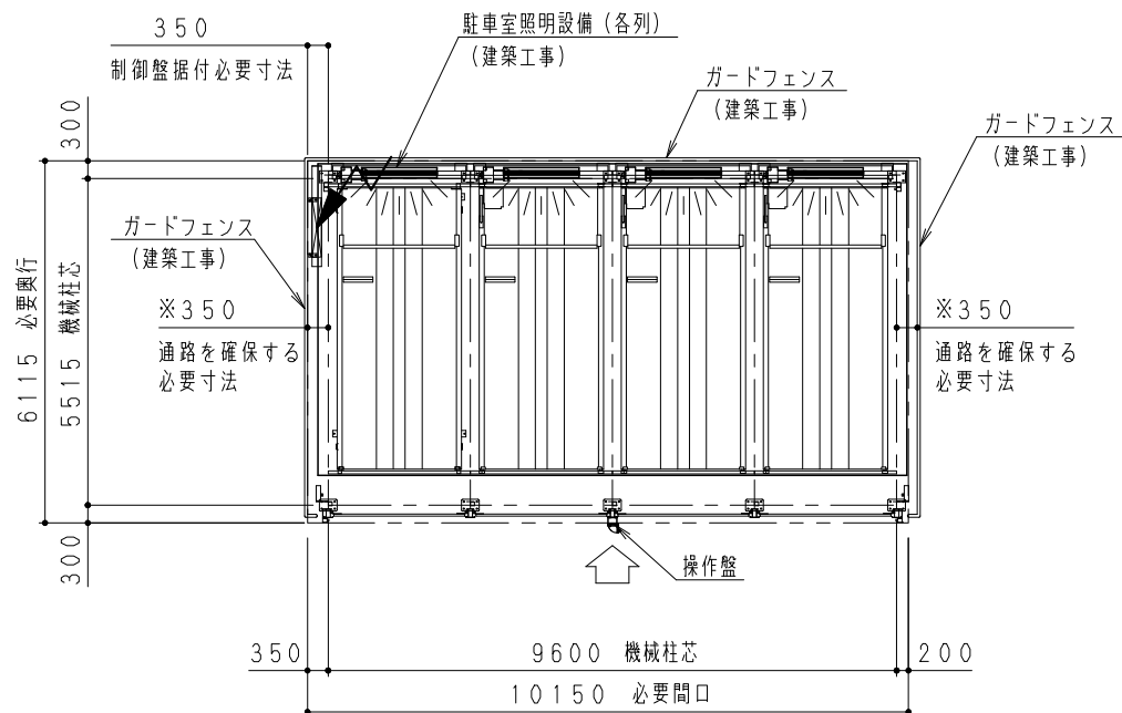
平面図
