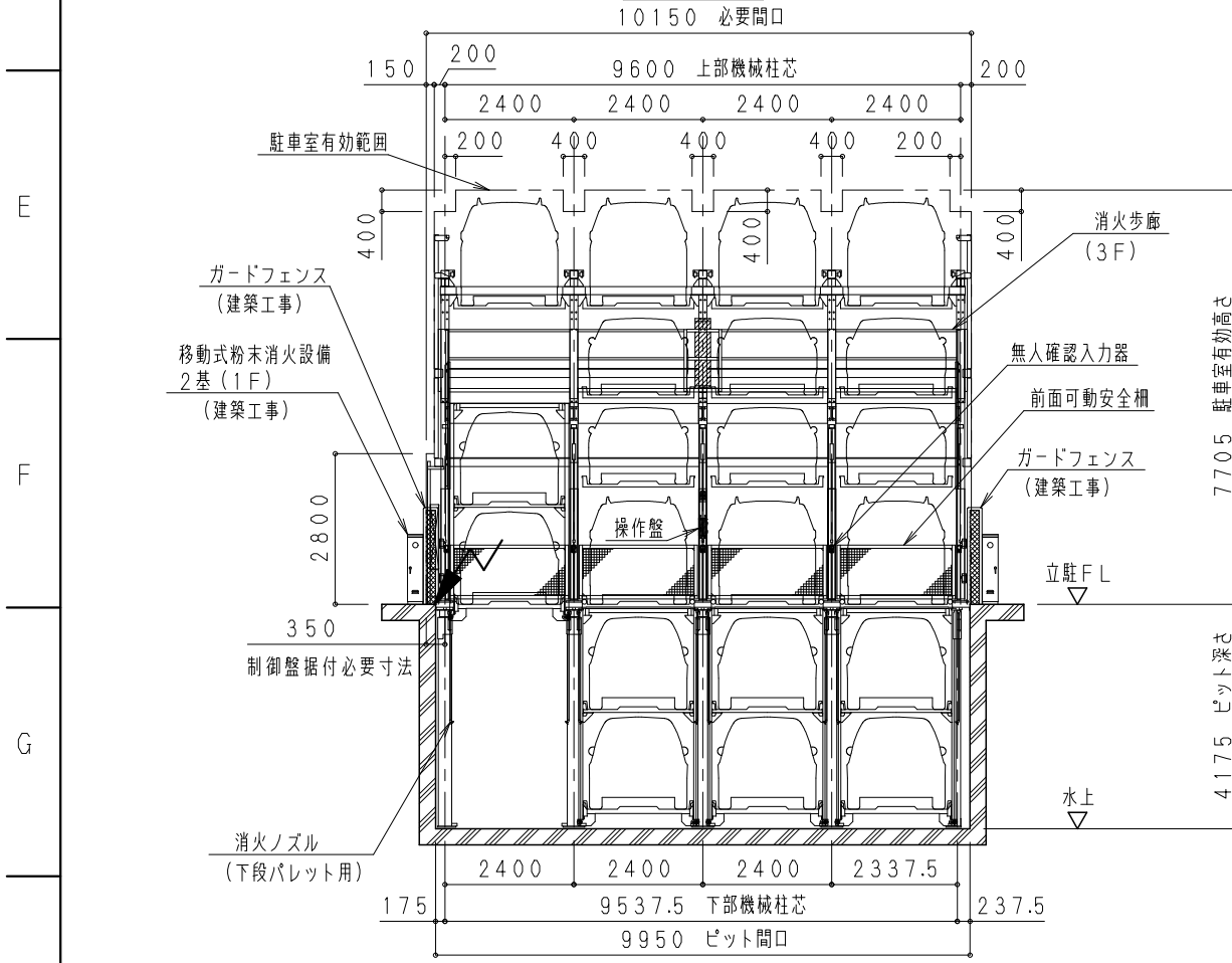
前列正面図
