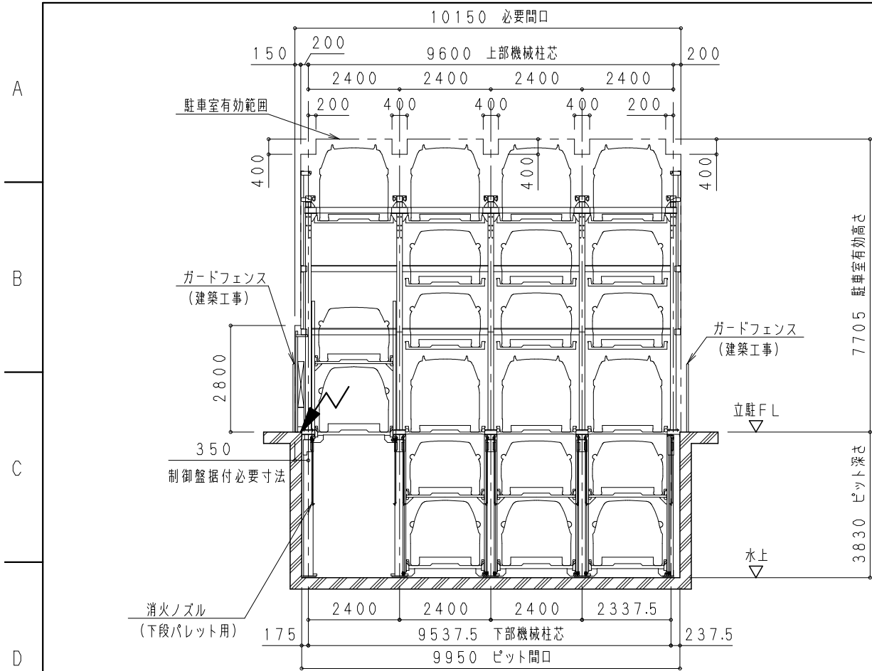
後列正面図
